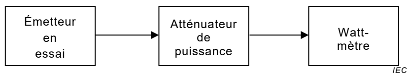
Figure 5 – Montage de mesure de la puissance de la porteuse
