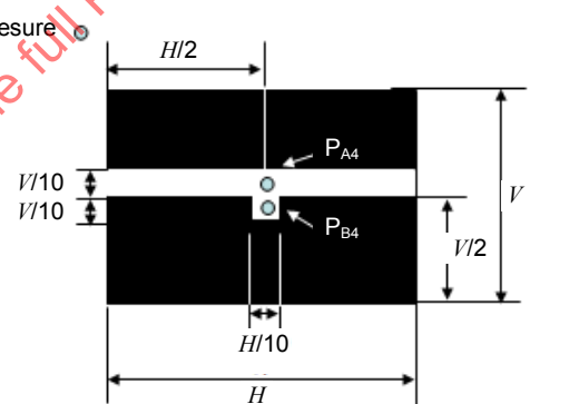
(d) APL faible – Mire L4
