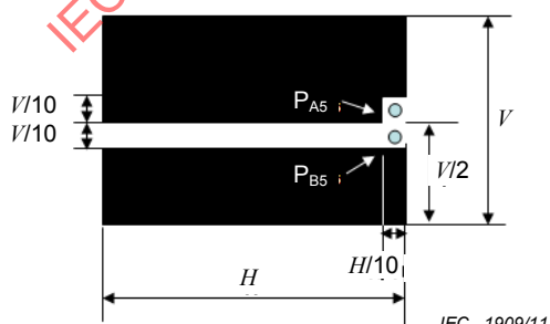
(e) APL faible – Mire L5
