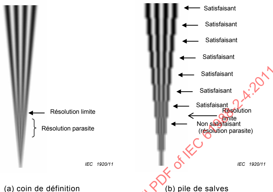
Figure 7 – Motif d'image pour l'évaluation de la résolution
