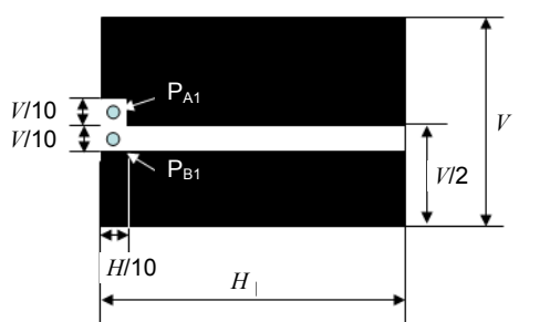
(a) APL faible – Mire L1
