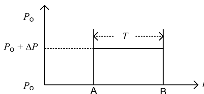
Figure 10 – Essai de réponse indicielle de la commande de puissance au niveau du redresseur
