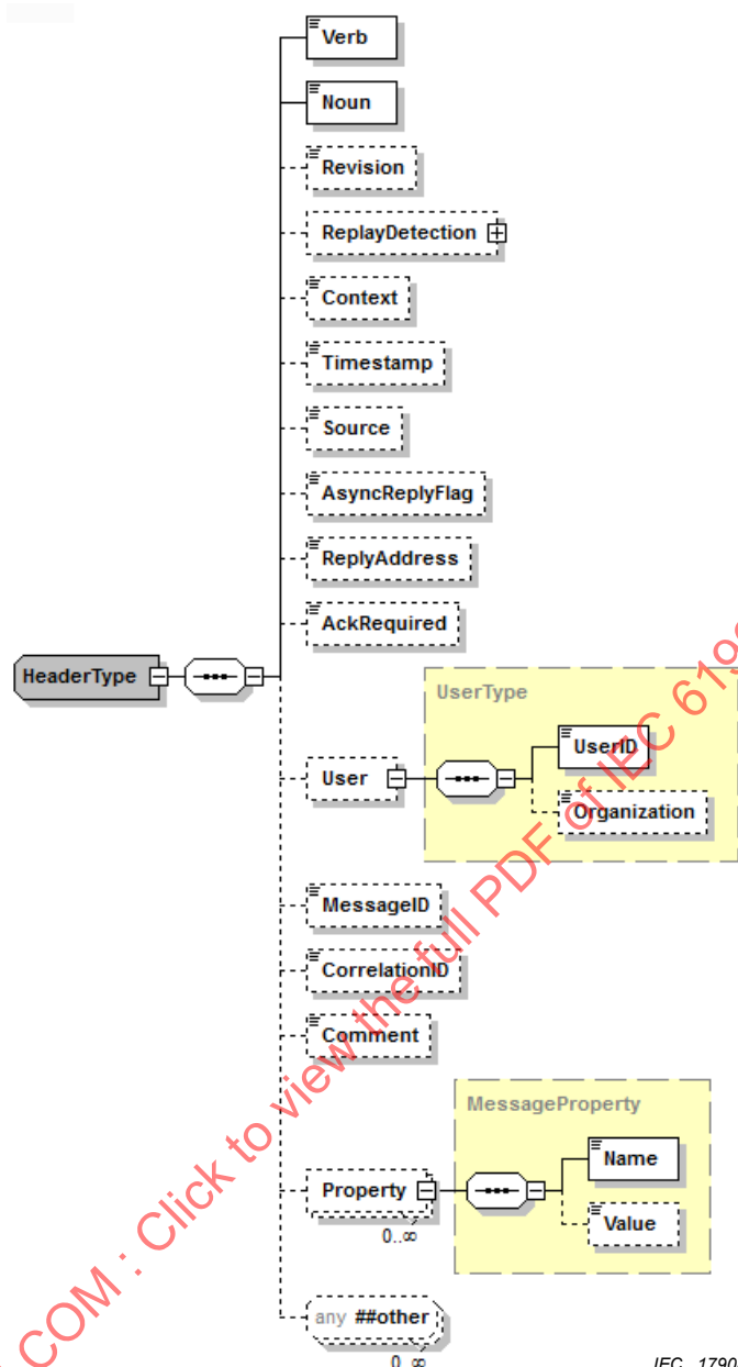
Figure 22 – Structure commune de l'en-tête de message
