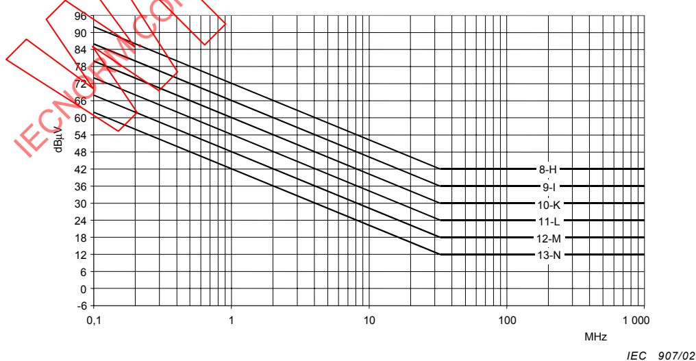
Figure C.2 – Méthode à 150 \Omega – Niveaux de référence pour perturbations conduites provenant de semiconducteurs (détecteur de crête)
