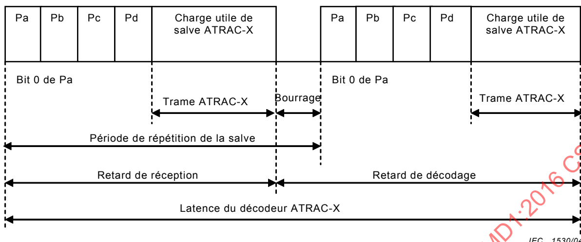
Figure 6 – Latence du décodage ATRAC-X
