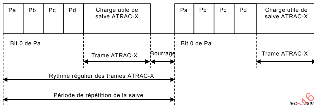
Figure 5 – Salve de données au format ATRAC-X
