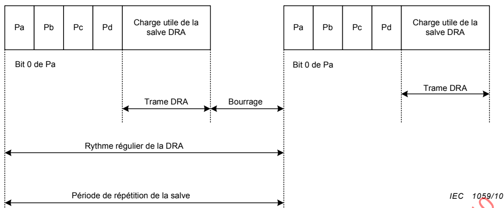
Figure 1 – Salve de données au format DRA
