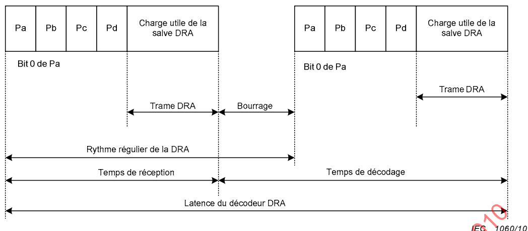
Figure 2 – Latence du décodage DRA
