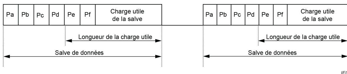
Figure 4 – Préambule de salve avec un préambule étendu
