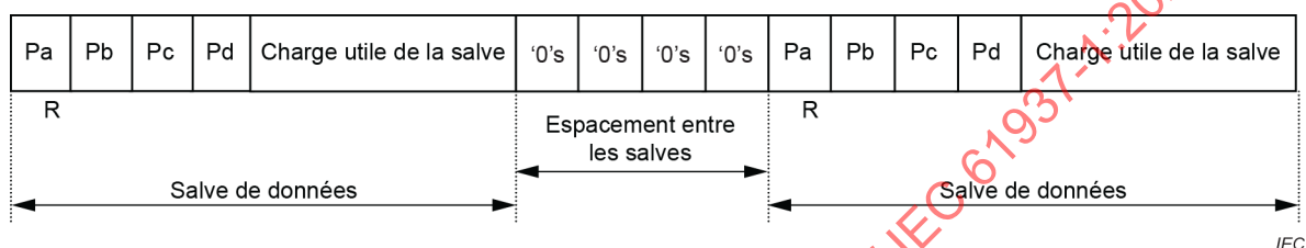
Figure 6 – Espacement entre les salves
