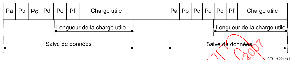
Figure 4 – Préambule de salve avec un préambule étendu
