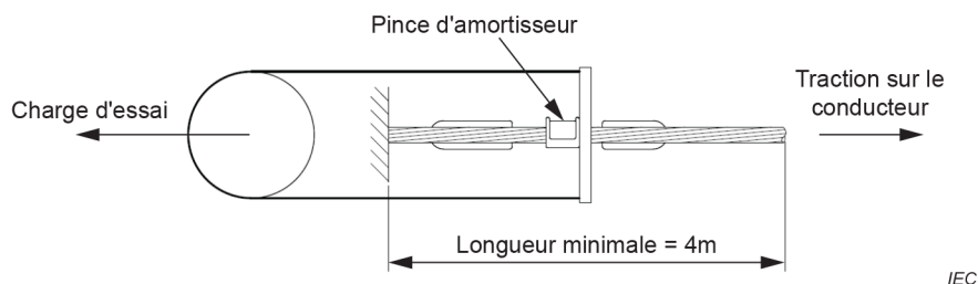
Figure 1 – Montage d'essai pour les essais de glissement longitudinal
