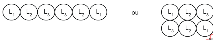
Figure 1 – Disposition recommandée pour l'installation des câbles unipolaires – Configuration plate
