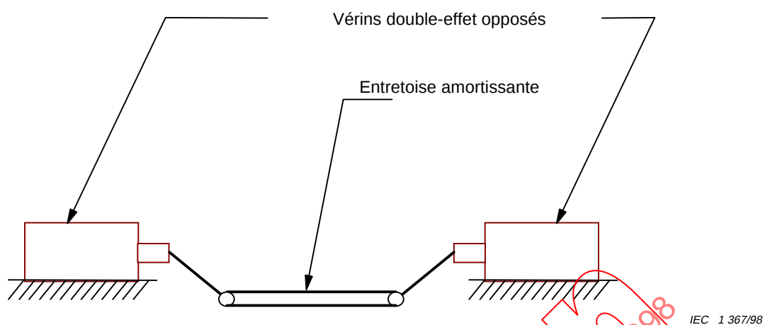
Figure 4 – Exemple de dispositif d'essai de compression et de traction
