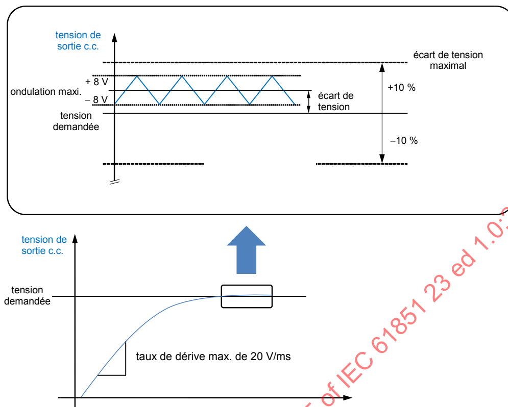
Figure 105 – Valeurs assignées maximales pour la dynamique de tension
