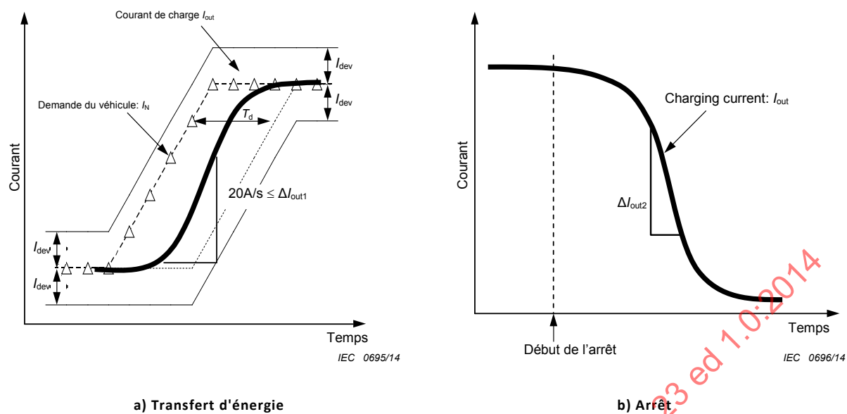
Figure AA.8 – Performance de réponse de sortie de la borne de charge à courant continu pour véhicule électrique
