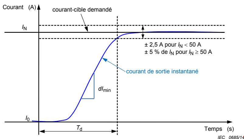
Figure 103 – Réponse à un échelon pour le contrôle de valeur constante
