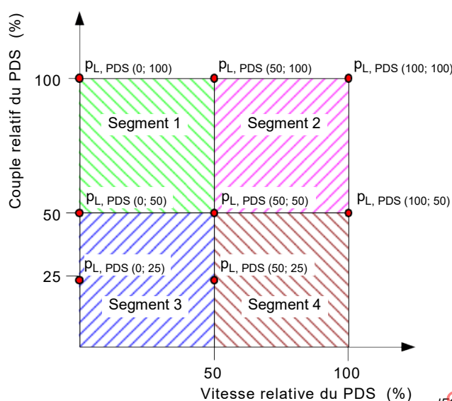
Figure 7 – Quatre segments de points de fonctionnement différents d'un PDS
