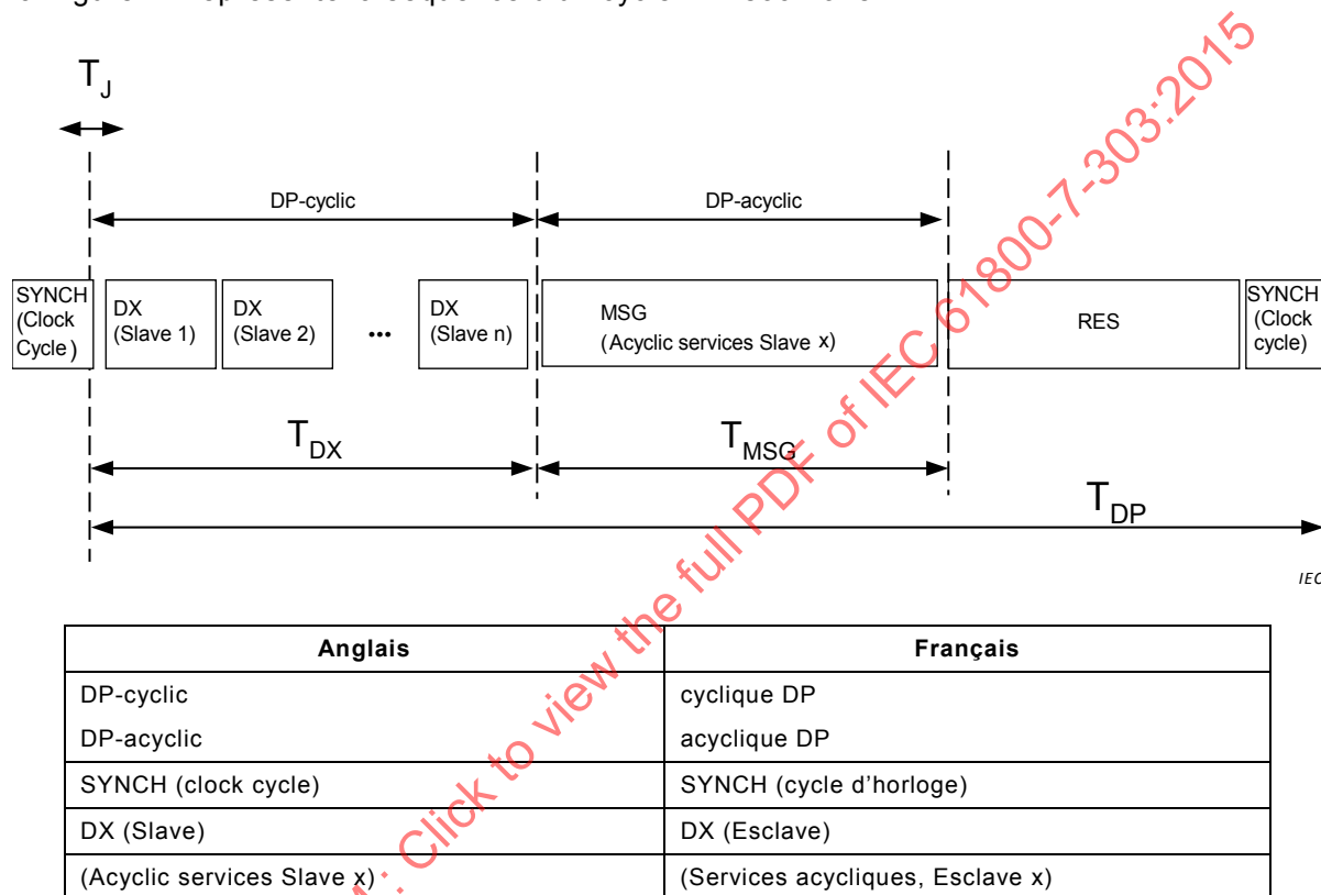
Figure 22 – Séquence d'un cycle DP isochrone
