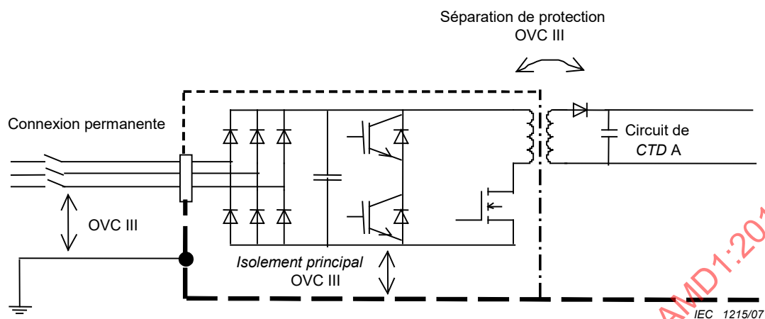
Figure B.13 – Evaluation de l'isolement pour les circuits accessibles de la CTD A
