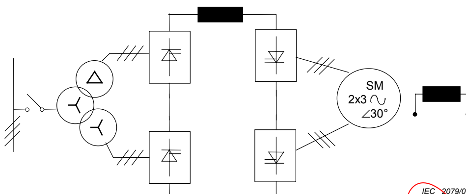
Figure 5 – Exemple de convertisseur à modules multiples et d'enroulements stator séparés
