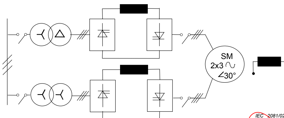
Figure 7 – Onduleur à commutation assistée par la charge (LCI) pour moteur synchrone en configuration partiellement redondante
