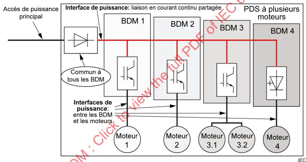
(b) Redresseur extérieur aux BDM
