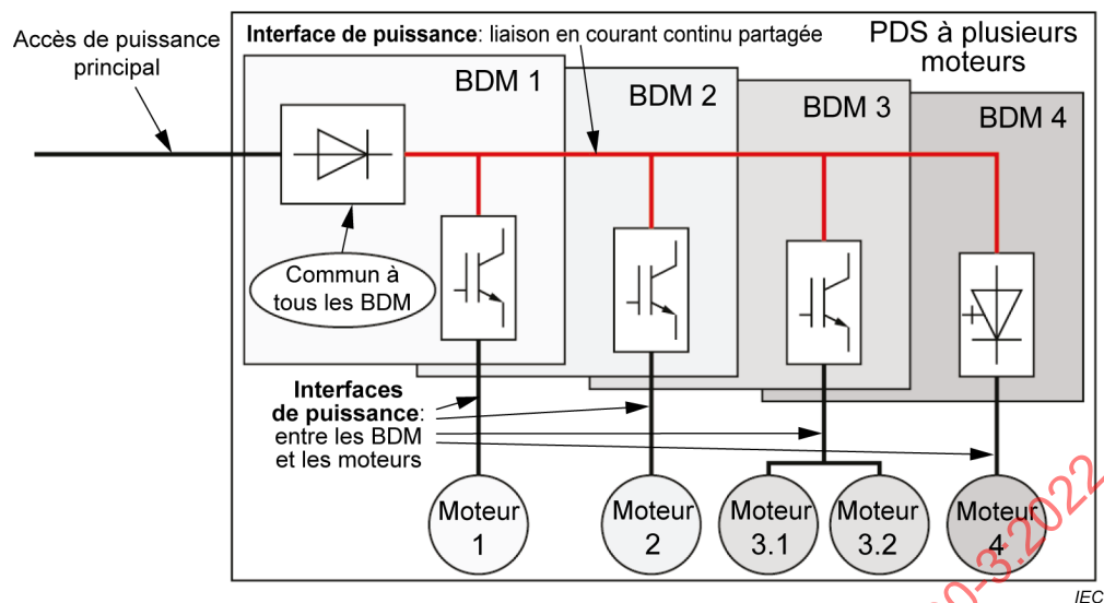
(a) Redresseur du BDM 1 alimentant plusieurs BDM
