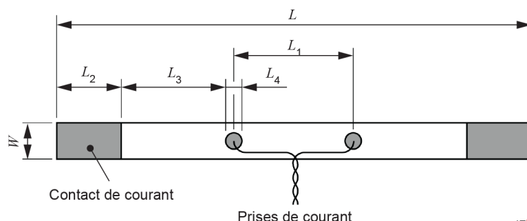
Figure 1 – Vue schématique d'un montage de mesure
