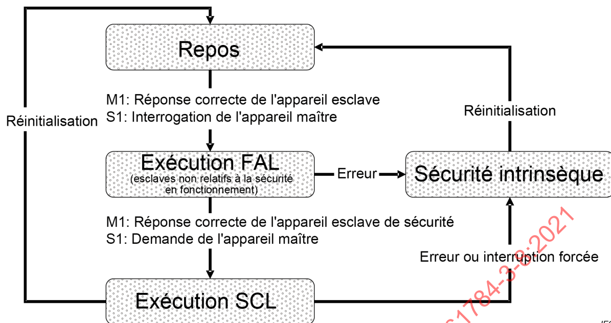
Figure 4 – Diagramme d'états
