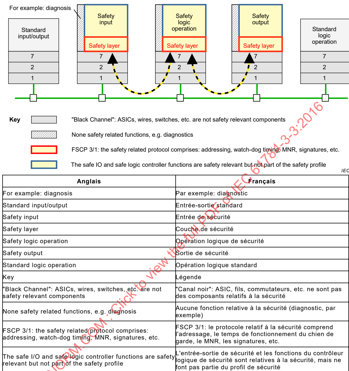
Figure 7 – Architecture de la couche de sécurité
