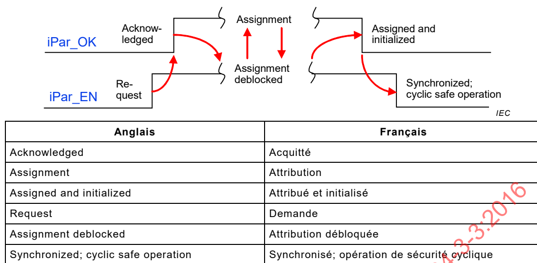
Figure 40 – Déblocage de l'attribution d'iParamètres par l'hôte F
