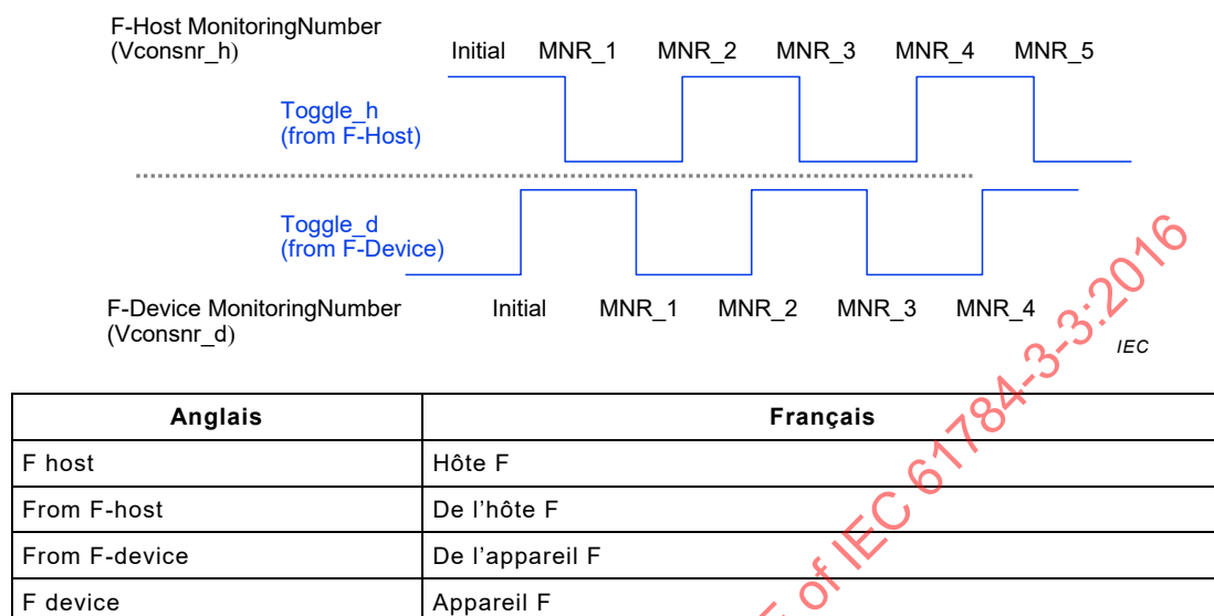
Figure 21 – Fonction du bit de basculement
