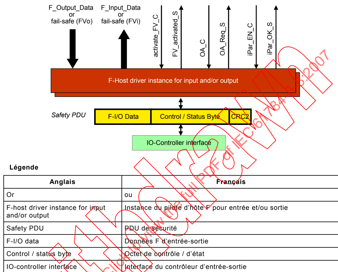
Figure 18 – Interface utilisateur F des instances du pilote de l'hôte F
