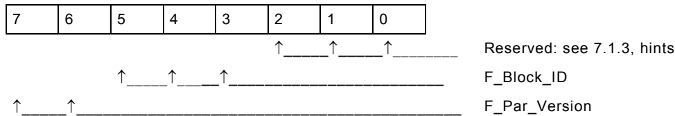
Figure 46 – F_Prm_Flag2
