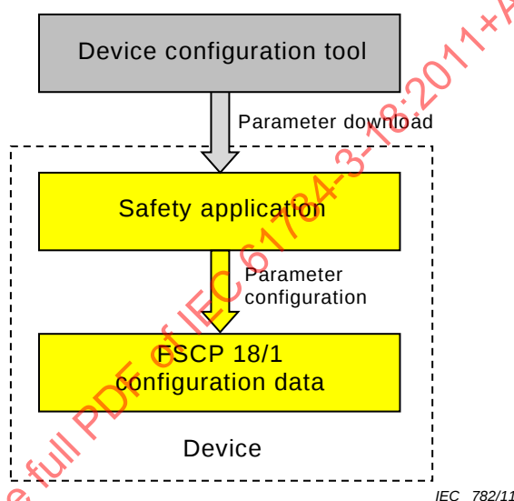
Figure 15 – Parameter handling
