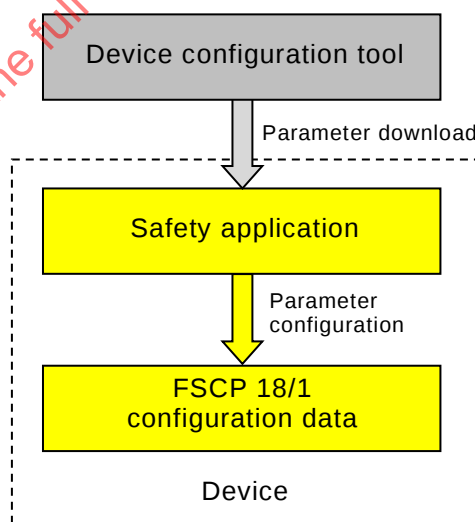
Figure 15 – Parameter handling
