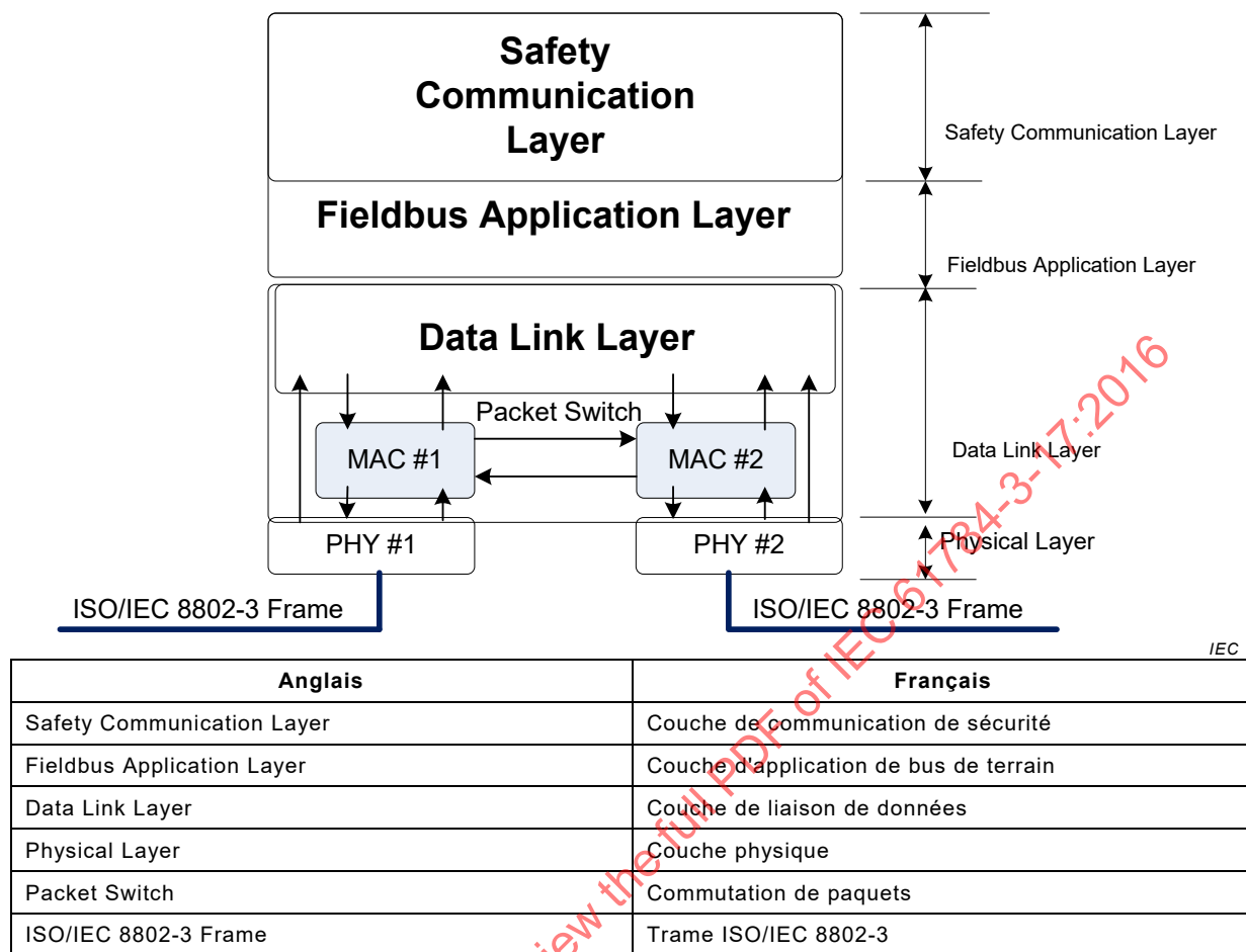
Figure 4 – Architecture de couche de sécurité
