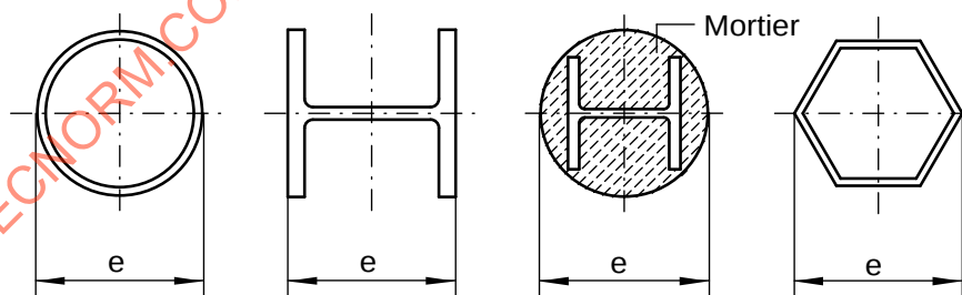
Figure 2e – Pieux
