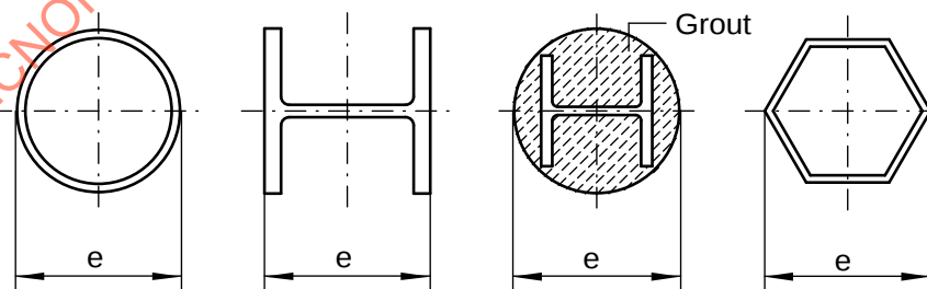
Figure 2e – Piles
