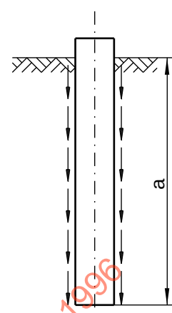
Figure C.3 – Réaction des structures élancées
