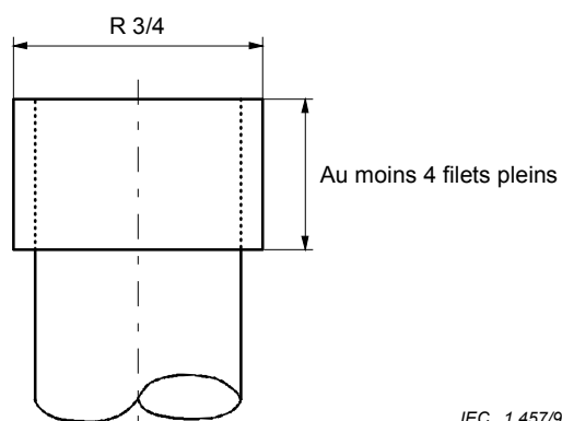
Figure 5 – Mandrin pour l'essai des écrous
