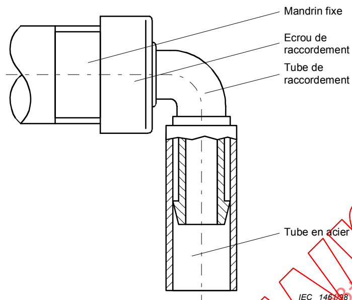
Figure 9 – Détail d'application du moment de pliure aux tubes de raccordement
