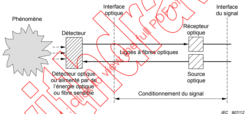
Figure 1 – Configuration d'un capteur à fibres optiques avec un détecteur passif et des lignes à fibres optiques distinctes pour les entrées et les sorties optiques
