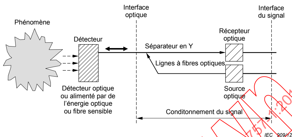
Figure 3 – Configuration d'un capteur à fibres optiques avec un détecteur passif et une ligne à fibres optiques pour les entrées et les sorties optiques; la séparation des signaux est réalisée par un séparateur en Y
