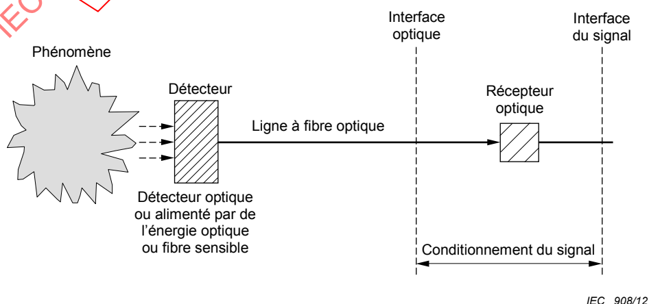
Figure 2 – Configuration d'un capteur à fibres optiques avec détection active
