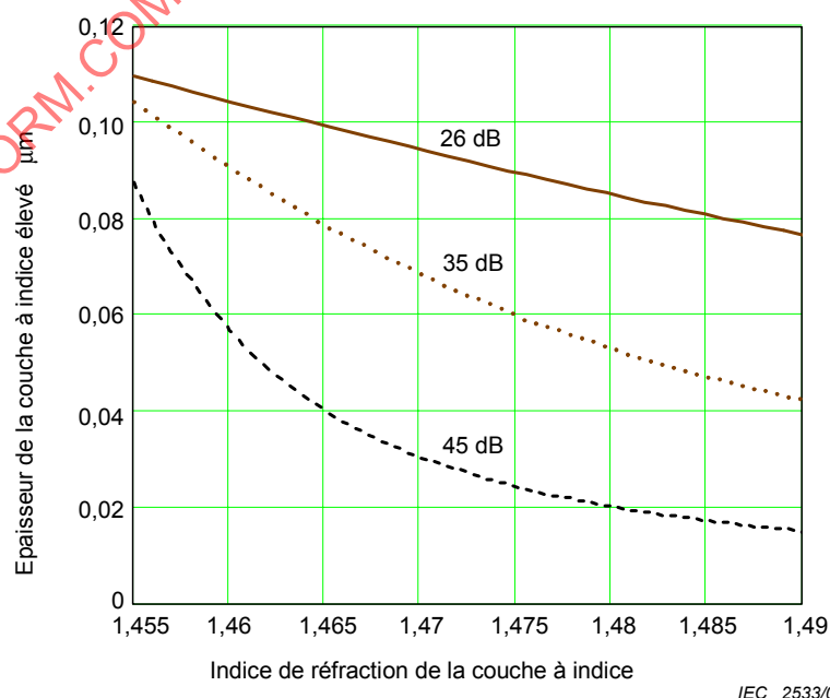
Figure 3 – Indice de réfraction de la couche à indice élevé et son épaisseur par rapport au facteur d'adaptation pour une fibre monomodale type à dispersion non décalée
