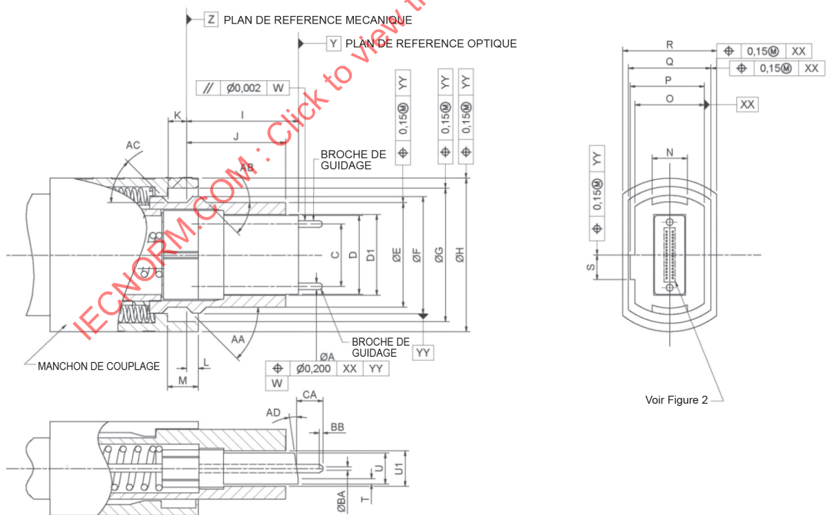
Figure 8 – Fiche mâle MPO, interface avec angle orienté vers le haut
