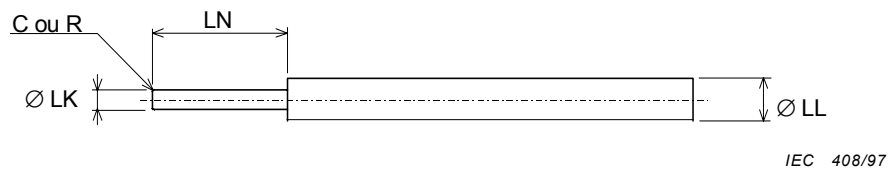
Figure 3b – Pointe de calibrage pour manchon d'alignement élastique
