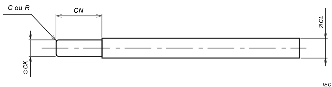
Figure 2 – Broche calibrée pour raccord
