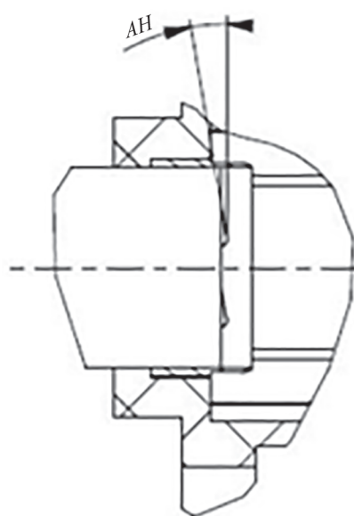
Figure 6 – Vue agrandie de la direction A (type APC)
