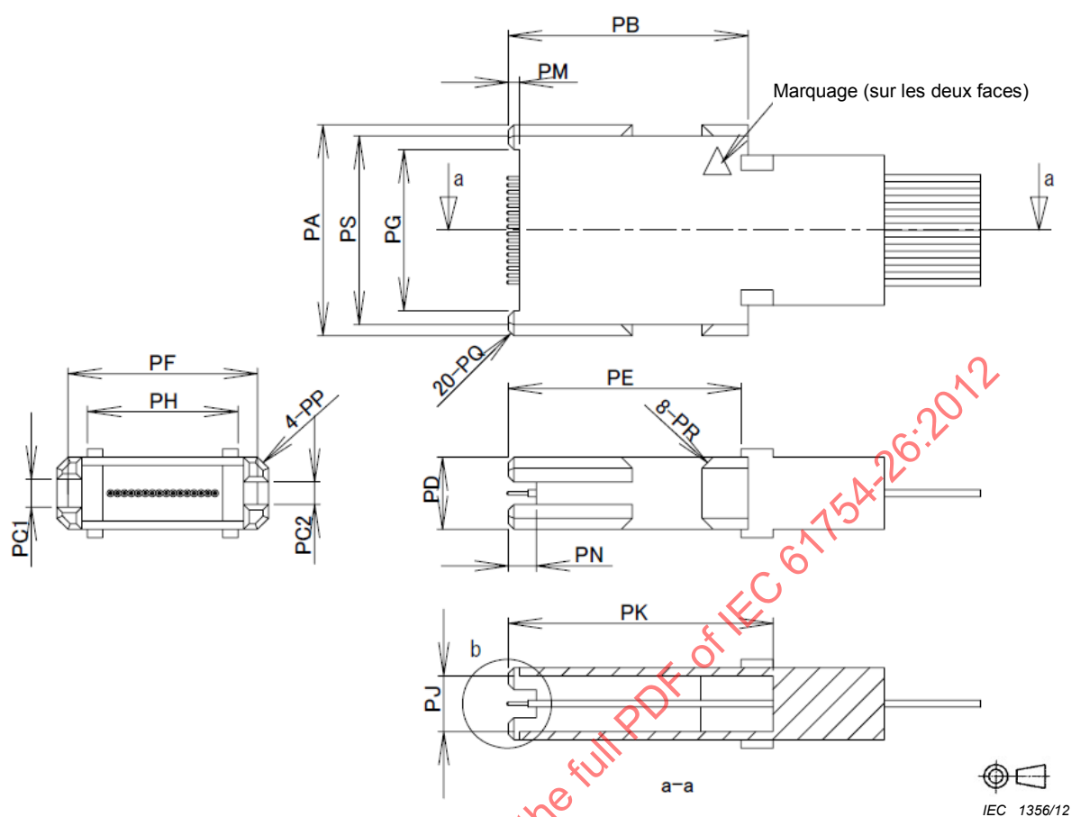
Figure 1 – Interface de connecteur mâle SF
