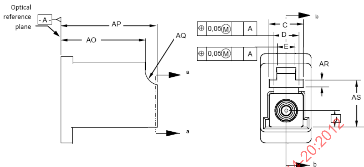
a) Dimensions de l'interface de connecteur intermédiaire simple
