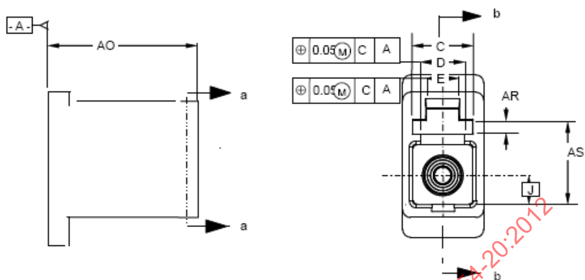
a) Dimensions de l'interface de connecteur intermédiaire Junior
