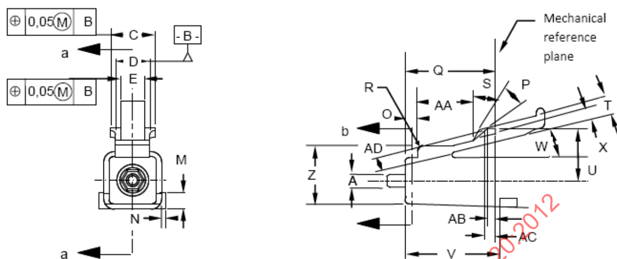
a) Interface de connecteur mâle
