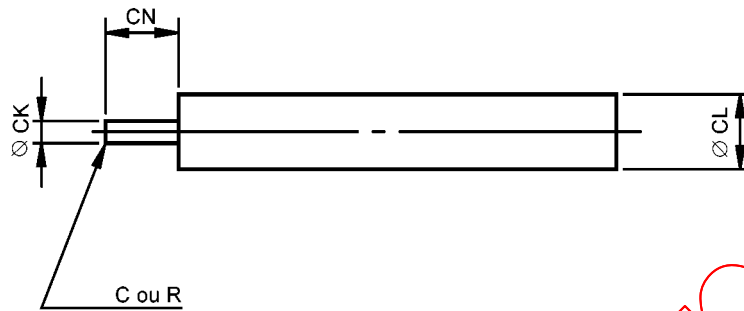
Figure 7 – Pointe de calibrage pour socle à dispositif actif
