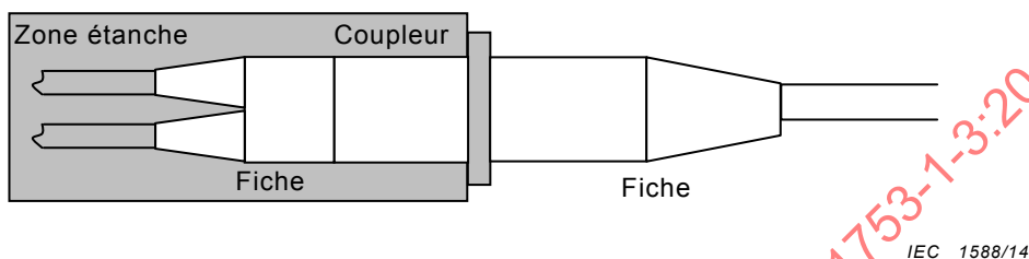
Figure 2 – Exemple de combinaison fiche-coupleur-fiche
