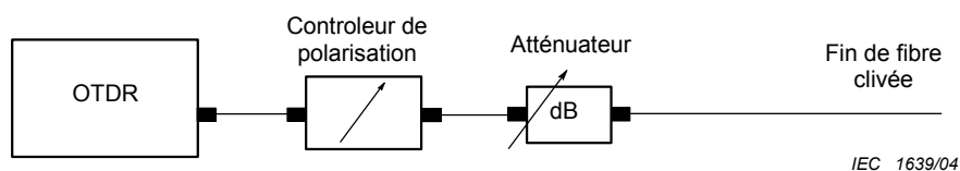
Figure 13 – Méthode de la réflexion pour l'essai de dépendance envers la polarisation des OTDR
