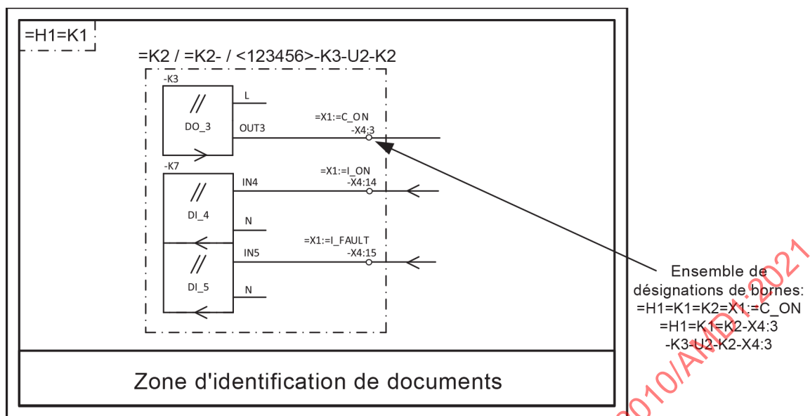
Figure 9 – Exemple de mise en œuvre de conception fondée sur la Figure 7 comportant des ensembles de désignations de bornes se rapportant aux aspects de fonction et de produit
