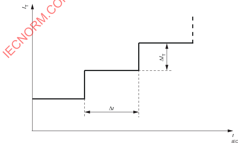
Figure 1 – Taille de pas maximale du courant d'essai continu lissé en augmentation ( I_T )
