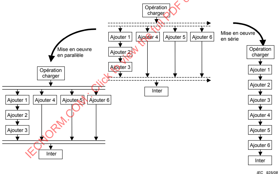
Figure 25 – Cheminements d'exécution alternatifs pour une exécution parallèle optionnelle
