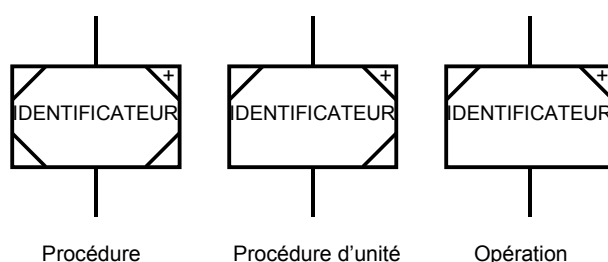
Figure 22 – Eléments procéduraux qui encapsulent des éléments procéduraux de recette d'un niveau inférieur
