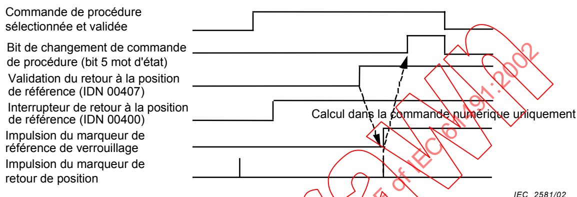
Figure 69 – Séquence de bits pour retour à la position de référence sous le contrôle de la commande numérique (cas 2.1)
