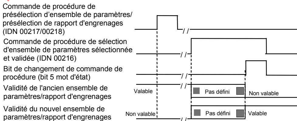
Figure 80 – Séquence de bits pour la commutation d'ensembles de paramètres et/ou du rapport d'engrenages
