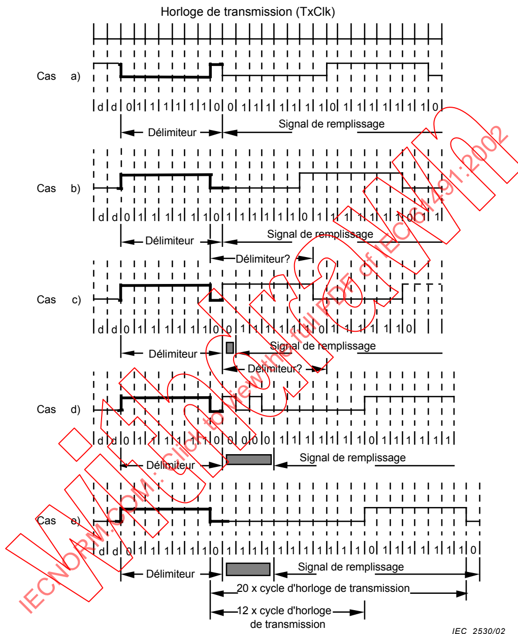
Figure 18 – Signaux de transmission corrects pendant les transitions de délimiteurs de message au signal de remplissage
