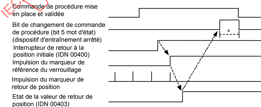
Figure 66 – Séquence des bits pour le retour à la position de référence commandée par le dispositif d'entraînement
