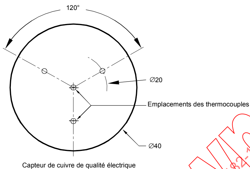
Figure 7a – Installation des thermocouples dans le calorimètre
