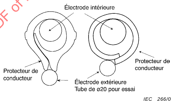
Figure 3a – Disposition de l'électrode extérieure pour essai d'épreuve A2
