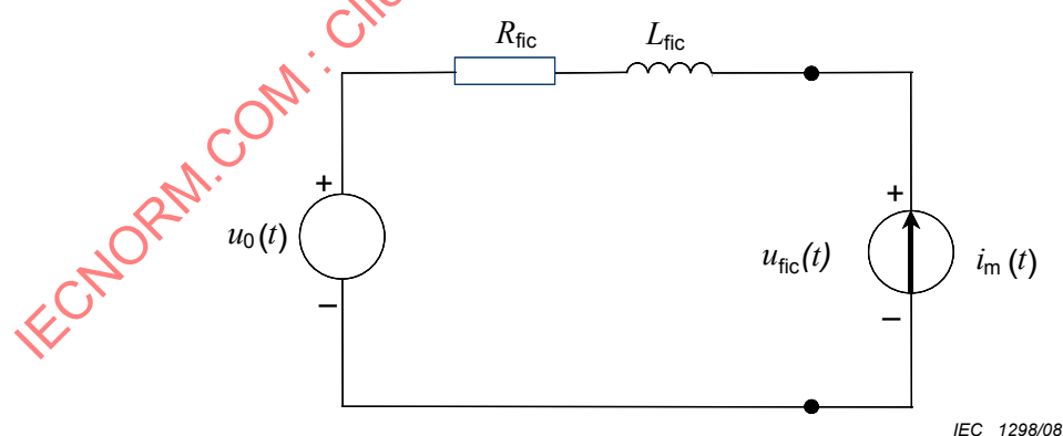
Figure 4 – Réseau fictif pour la simulation d'une tension fictive
