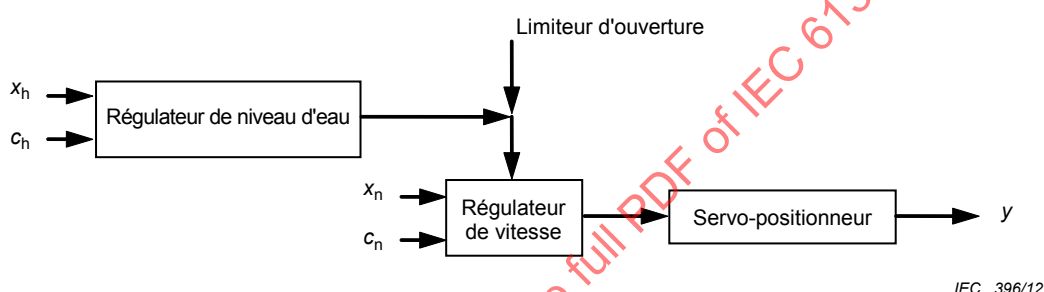
Figure 14 – Système de régulation avec régulateurs de niveau et de vitesse en série
