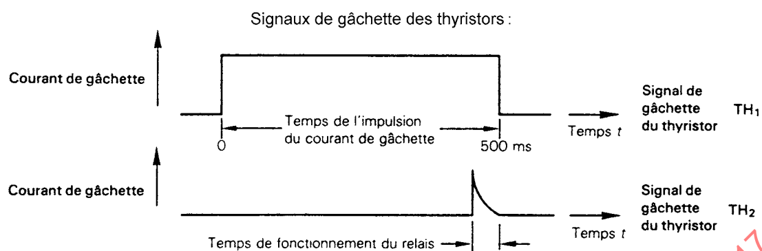
b) Comportement temporel des thyristors TH 1 and TH 2
