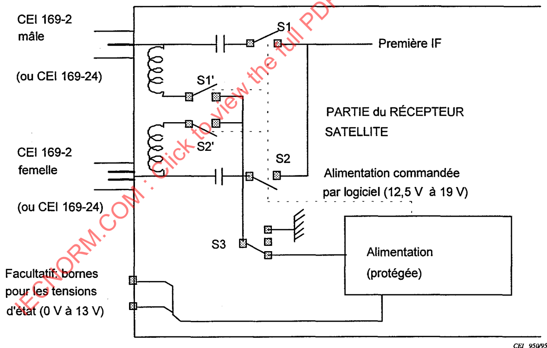
Figure 3 – Interface de la sortie première FI du LNB avec l'entrée du récepteur (le schéma est indiqué à titre d'exemple )
