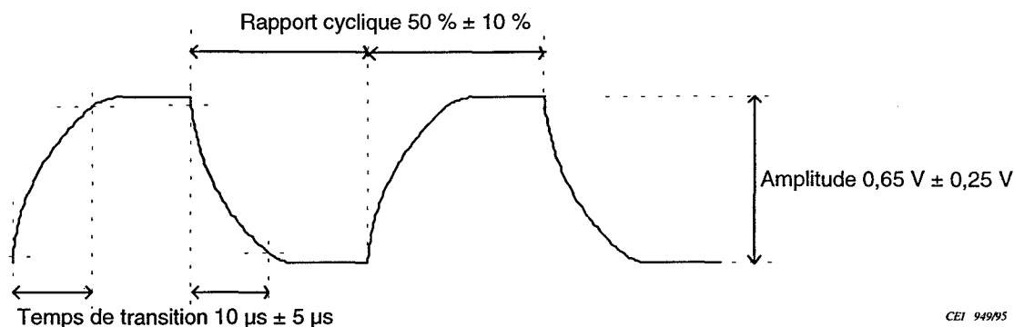
Figure 2 – Signal de commande superposé à la tension d'alimentation pour le commutateur de polarisation combiné à un convertisseur double bande
