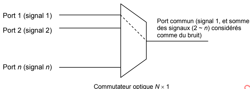
Figure 1 – Diaphonie pour commutateur optique N \times 1
