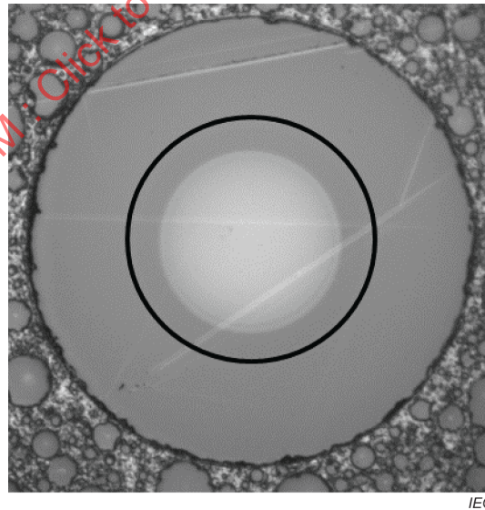
Figure B.2 – Exemple 2 de défauts et d'éraflures
